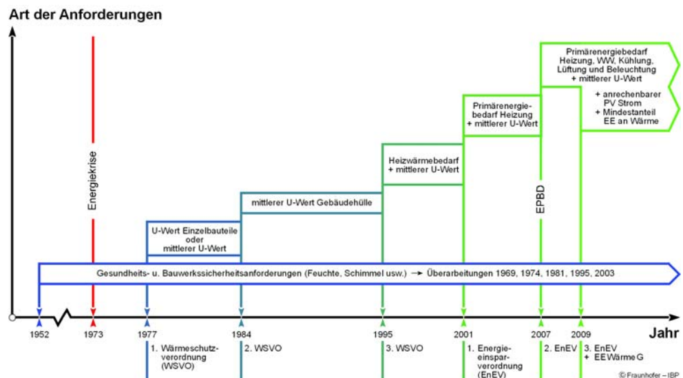
Bild 1: Übersicht über die Entwicklung der Anforderungen an das energiesparende Bauen in den letzten 60 Jahren
